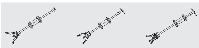
Extrator com duas Garras Interior
